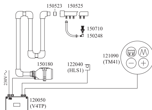
10 120050 V4TP elektronika v zapojení pro spínání kompresoru s pulsací a regulací otáček vč. hladinového snímače HLS1 a možnosti automatického vysoušení. 120045 V4T control electronics wired for blower switching with pulsation and speed regulation incl. water level sensor HLS1 for dry run protection and pos.
