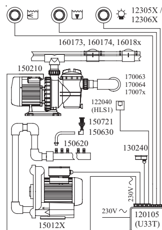
12 120105 elektronika U33T ovládaná piezo a mikrozdvihovými tlačítky 120105 control electronic U33T controlled with piezo and micro-lifting buttons
