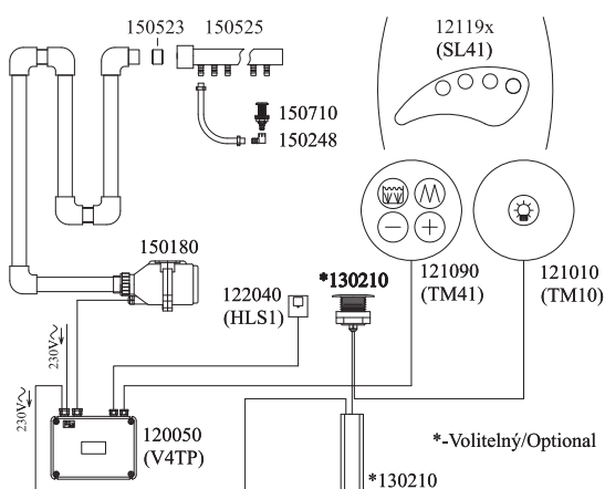
11 120056 V5TP elektronika v zapojení pro spínání kompresoru s pulsací a regulací otáček a osvětlení (halogen nebo LED CoolLight) vč. hladinového snímače HLS1 a možnosti automatického vysoušení. 120045 V4T control electronics wired for blower switching with pulsation and speed regulation and light (halogen or LED CoolLight) incl. water level sensor HLS1 for dry run protection and pos. automatic drying.
