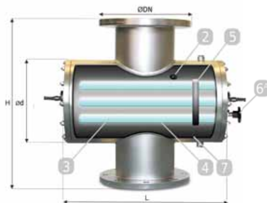
2 - Teplotní senzor/Temperature sensor 3 - UVM lampa/UVM® lamp 4 - Křemenné pouzdro /Quartz sleeve 5 - Pohon stěrače/Wiper mechanism 6 A – Ruční stěrač/Manual wiper 7 - Komora UV lampy z nerezové oceli 316L s leštěným vnitřním povrchem/ 316L stainless steel UV reactor with polished internal surface
