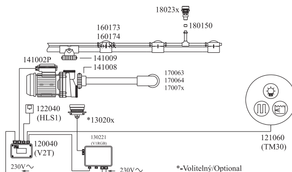
8 120040 V2T elektronika v zapojení pro spínání čerpadla a chromoterapie 13020x s elektronikou V1RGB nebo chromoterapie 130210 s integrovanou elektronikou v těle světla s jističím proti chodu naprázdno hladinovým snímačem HLS1. 120040 V2T control electronics wired for pump and chromotherapy switching 13020x with V1RGB electronics or chromotherapy 130210 with electronics integrated into the light with HLS1 water level sensor for dry run protection.
