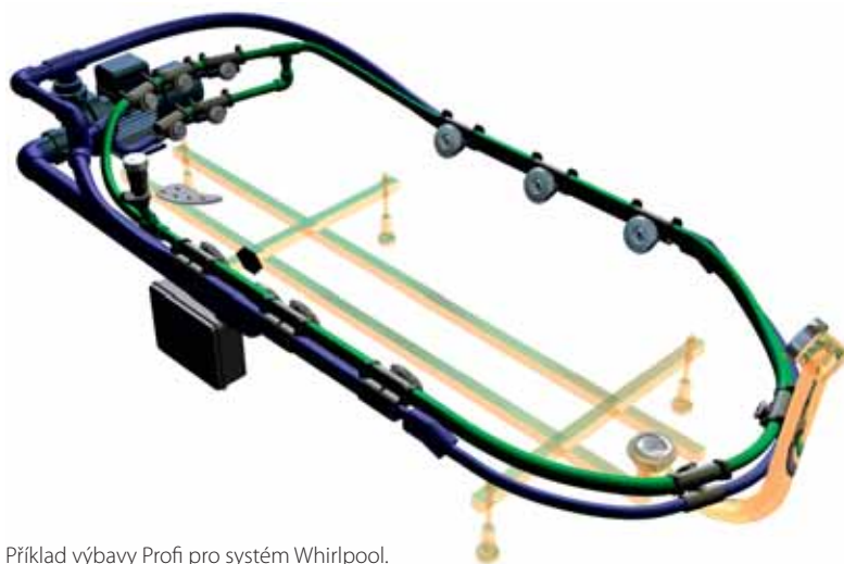
Příklad výbavy Profi pro systém Whirlpool. Example of Profi equipage for Whirlpool system.
