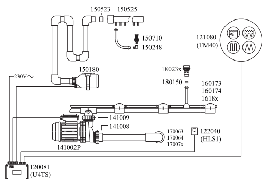
9 120081 U4TS elektronika v zapojení pro spínání čerpadla a kompresoru s pulsací a jističím proti chodu naprázdno hladinovým snímačem HLS1. 120081 U4TS Control electronics wired for pump and blower switching with pulsation and HLS1 water level sensor for dry run protection.
