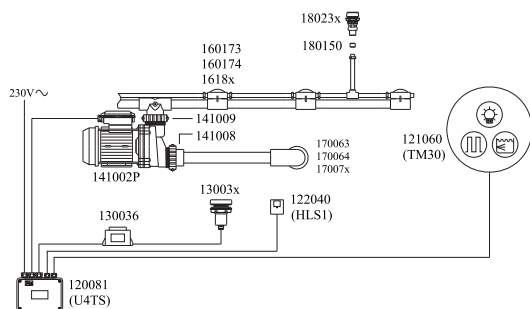
7 120081 V4TS elektronika v zapojení pro spínání čerpadla a osvětlení (halogen nebo LED CoolLight) s jističím proti chodu naprázdno hladinovým snímačem HLS1. 120046 V4TS control electronics wired for pump and light (halogen or LED CoolLight) switching with HLS1 water level sensor for dry run protection.
