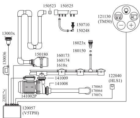
17 120057 V5TPH elektronika v zapojení pro spínání čerpadla a kompresoru s pulsací, regulací otáček kompresoru, osvětlením (halogen nebo LED CoolLight), jističným proti chodu naprázdno hladinovým snímačem HLS1 a možnosti automatického vysoušení. 120057 V5TPH control electronics wired for pump and blower switching with pulsation, blower speed control, light (halogen or LED CoolLight), water level sensor HLS1 for dry run protection and pos. automatic drying.
